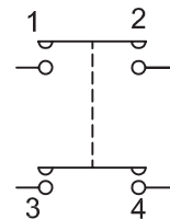
CIRCUIT DPST
